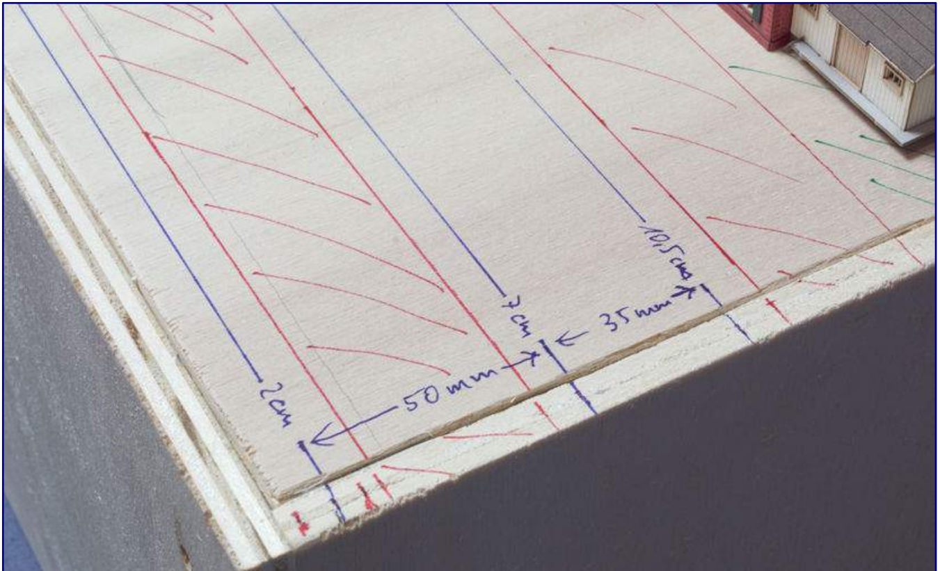
Sobald die obere Ebene montiert werden kann, erfolgt das Anzeichnen der Bahnsteig- und Gleislage sowie das Festhalten wichtiger Maße für die weiteren Arbeiten.
