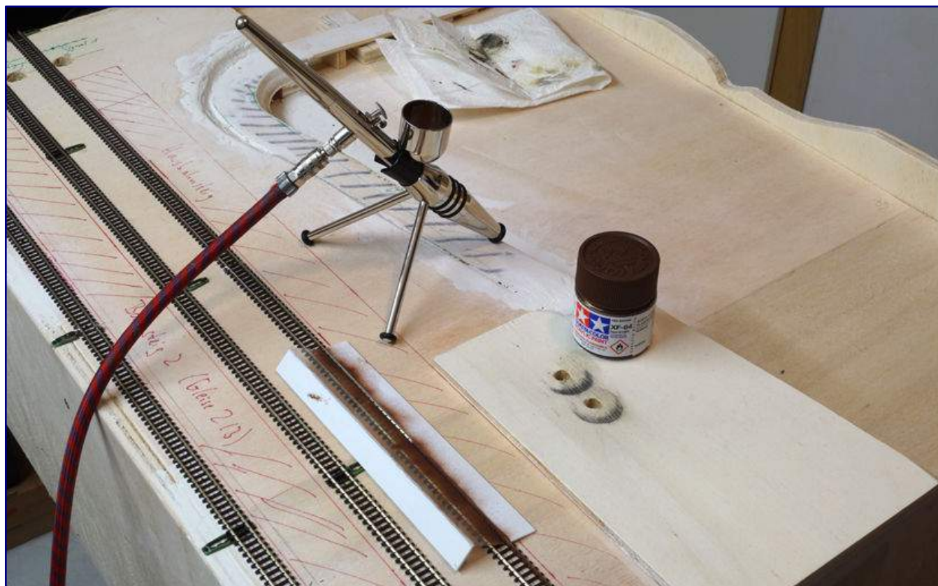
Die Schienenflanken erhalten mit Tamiya-Farbe und dem Spritzapparat eine Rost-Patina. Um einen Farbauftrag an unerwünschten Stellen vorzubeugen, bedienen wir uns einer selbstgebauten Sprühschablone aus Polystyrol-Teilen.
