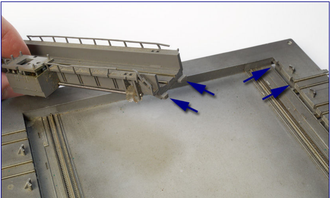
Die Pfeile im Bild kennzeichnen die Führungsnasen an der Bühne (links) und die zugehörigen Aussparungen an einem Grubenende (rechts), erkennbar am dort fehlenden Gleisabgang, die das Herausnehmen in gekipptem Zustand ermöglichen.
