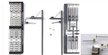
471) ZB471 (Zm)
