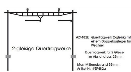
482) ZF482
